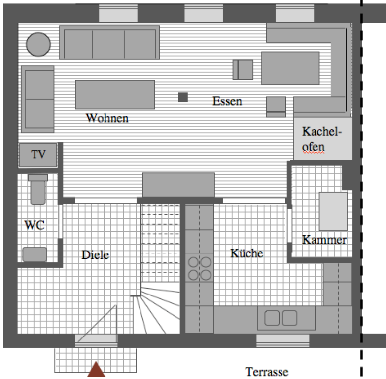
Grundriss ehemaliger Kälberstall: Erdgeschoss
